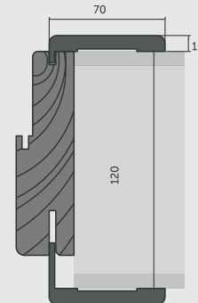
Máxima apertura contramarco
