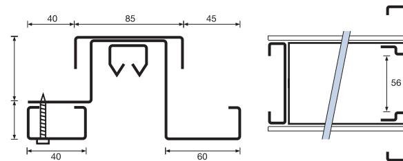
SECCIÓN PERFIL Y RIEL
