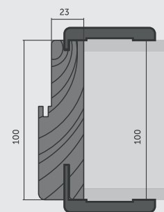
Mínima apertura contramarco
